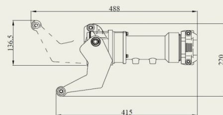
PC4, размеры ± 5мм
