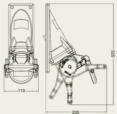
PC2, размеры ± 5мм
