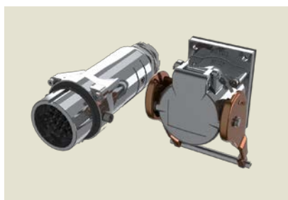
PC2, вилка и панельная розетка, тип «пушпульный»
