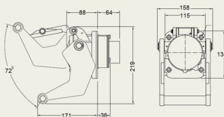
PC4, размеры ± 5мм
